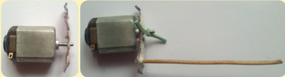
Gambar 2.30. Pemasangan tutup botol dan lidi pada Motor Listrik DC.
